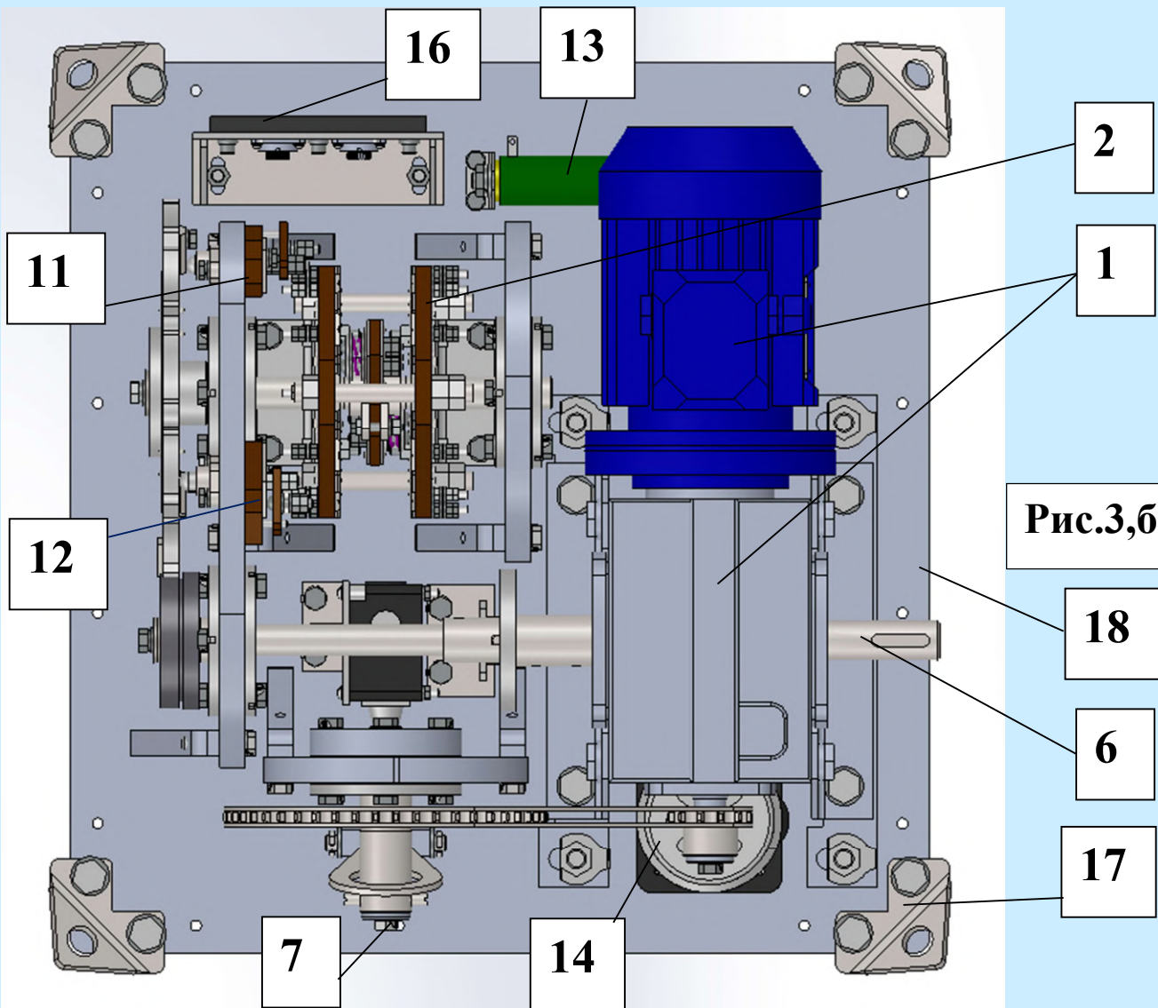
Рис.3 - Приводной механизм ПМ-ПБВ правый без кожуха
